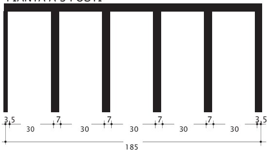
PIANTA A 5 POSTI
