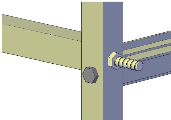
NODO MONTANTE CON PROFILO ANTERIORE
