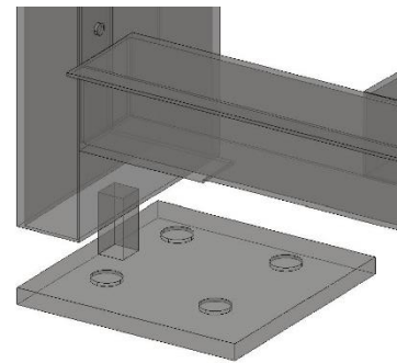
PIASTRA DI FISSAGGIO REGOLABILE IN ALTEZZA
